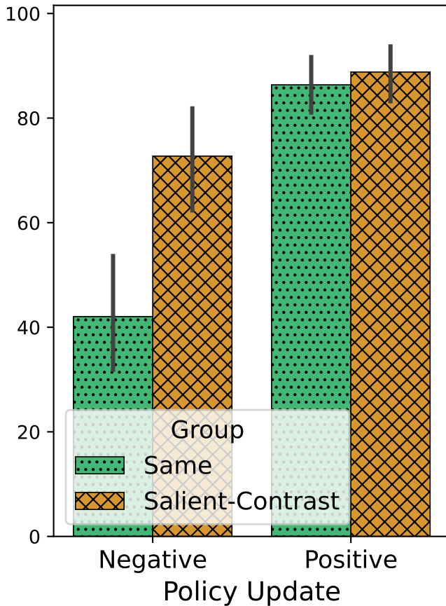
Minigrid
